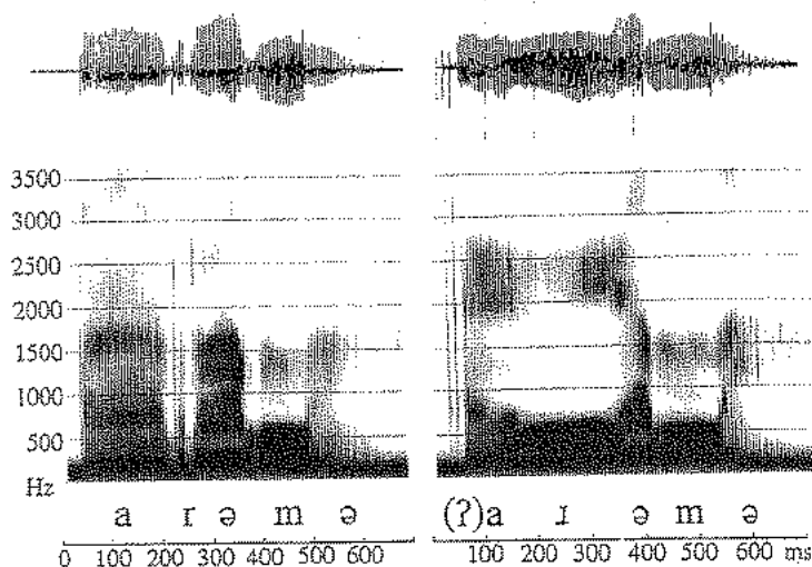
Figure 7.23 Waveforms and spectrograms of the Eastern Arrernte words arəmə [arə h mə] 'louse' and arəmə [ʔarə h mə] 'sees' illustrating the contrasting rhotics of the language. (Note the voiced stop-like onset to the nasals, see chapter 4.)
